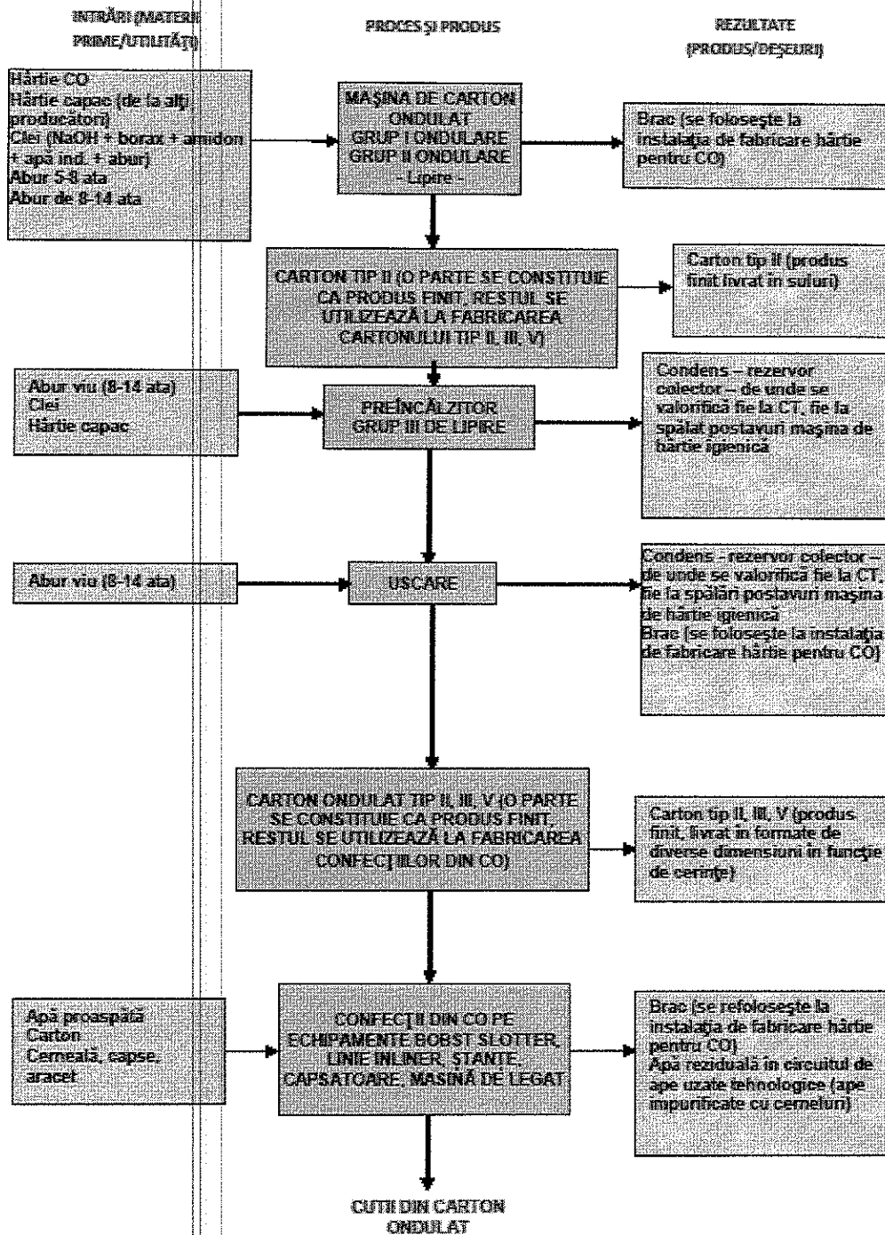
Fig. 4 INSTALAȚIA DE FABRICARE CARTON ONDULAT ȘI CONFECȚII DIN CARTON ONDULAT
